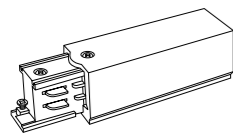
ST030.409.10R ■ черный ST030.509.10R □ белый правый токоподвод для трехфазного шинопровода L109 × W34 × H17 MM
