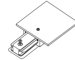
ST012.479.00 ■ черный ST012.579.00 □ белый ввод питания для однофазного встраиваемого шинопровода L117 × W60 × H18 MM
